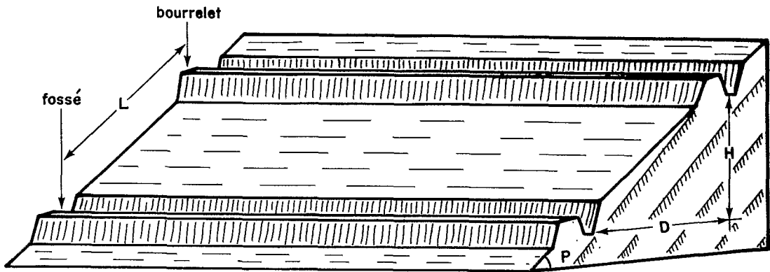
Vue perspective d'un réseau de banquette
