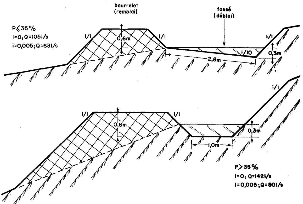
Profil en travers d'une banquette
