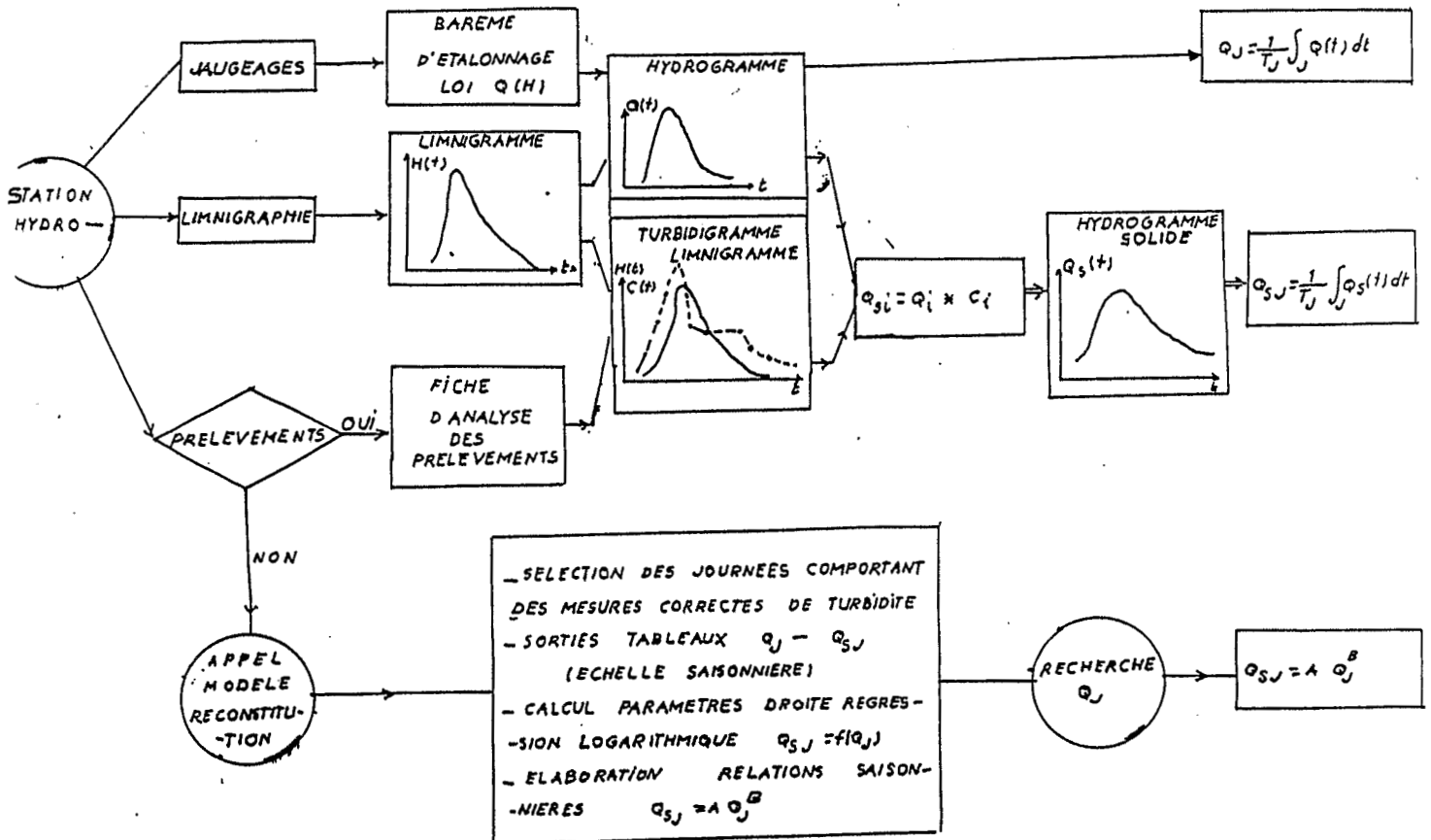
Fig 8 : Détermination d'un débit solide moyen journalier.
