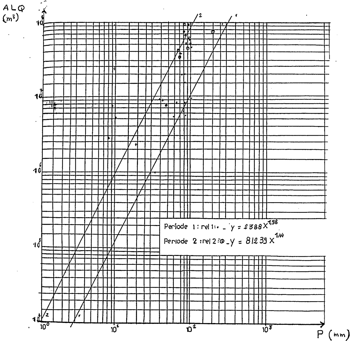
Fig 9 : Relations saisonnières pluie-apport liquide.
