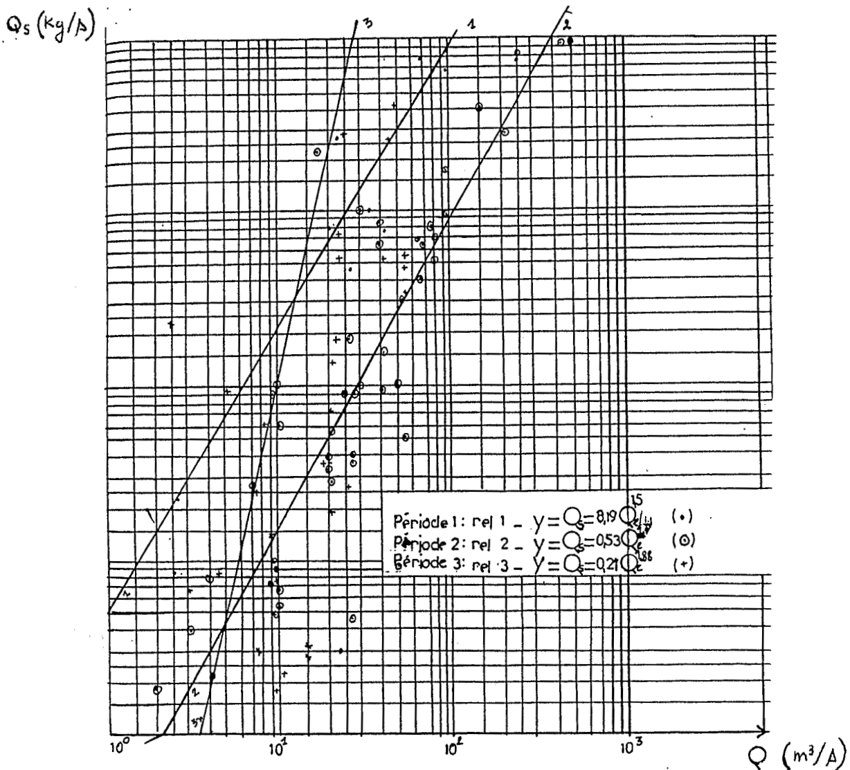
Fig 11 : Relations saisonnières débit solide-débit liquide.
