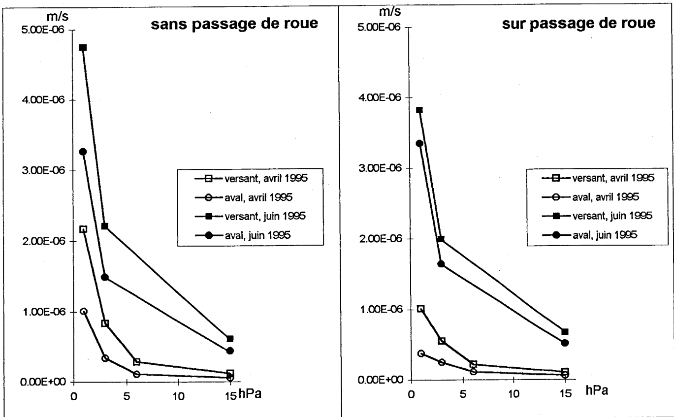
Figure 3 - Conductivité hydraulique (m/s) en fonction de la succion (hPa) Comparaison sur et hors passage de roue, début (juin) et fin (avril) de cycle cultural, et entre le versant et l'aval.
