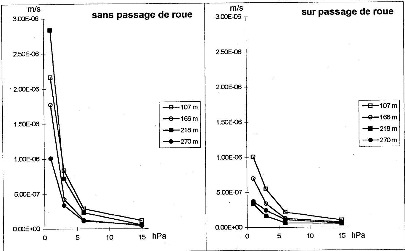
Figure 2 - Conductivité hydraulique (m/s) en fonction de la succion (hPa) Comparaison sur et hors passage de roue, en fonction de la distance amont. Mesures d'avril 1995, en fin de cycle cultural
