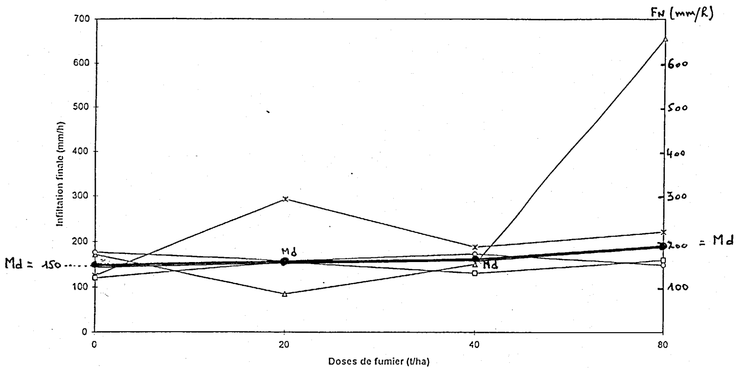
Figure 1. Effet de différentes doses de fumier sur l'infiltration finale mesurée à l'arroiseur manuel dans les sols de coteaux maigres de Verrières. (FN médians en mm/h)
