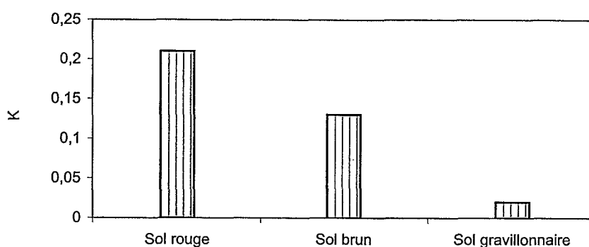
Figure 5 : Erodibilité K des sols d'après les érosions mesurées en 1998
