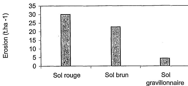
Figure 4 : Erosions (t/ha/an) mesurées sur parcelles nues (campagne 1998)
