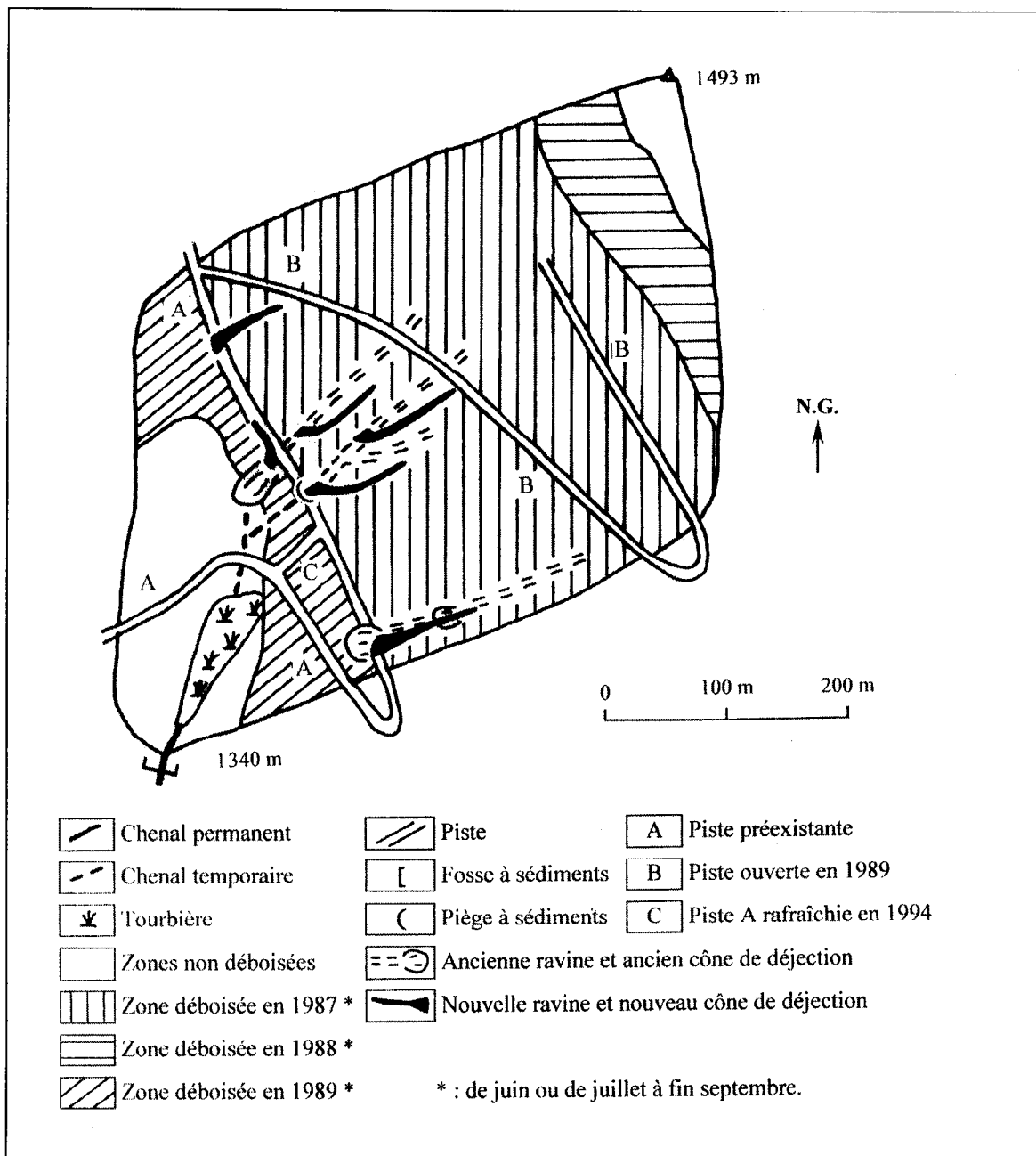
Figure 2 - Présentation du bassin versant de la Latte.
