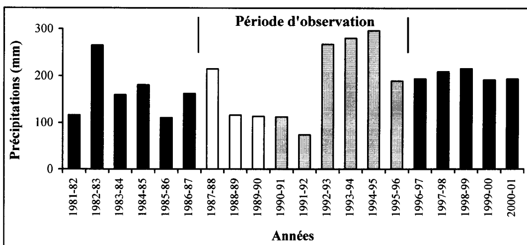
Figure 5 - Précipitations journalières maximales sur le bassin versant de la Latte.
