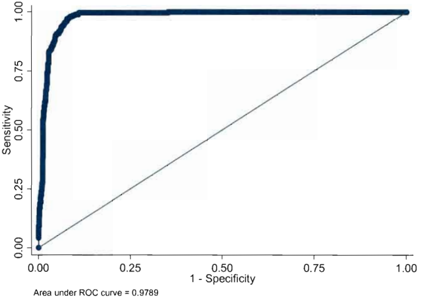
Graphique 7: Courbe ROC du pouvoir prédictif total du modèle
