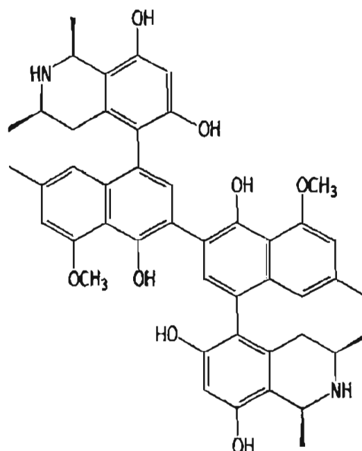
Figure 27 : Structure de la Michellamine B [67]
