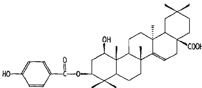
Figure 32 : Structure de l'acide 3-p-hydroxybenzoate 1 \beta -hydroxyaleuritolique [67]
