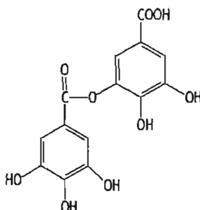
Figure 43 : Structure de l'acide digallique [67]
