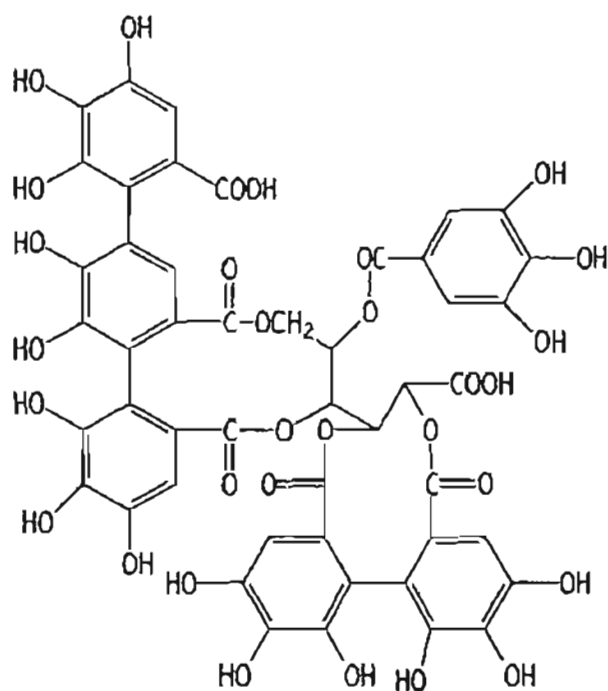
Figure 44 : Structure de la Shephagénine A [67]
