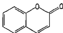
Figure 36 : structure de la benzo \alpha -pyrone
