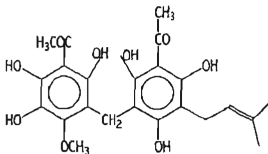
Figure 46 : Structure de Mallotojaponine [74]
