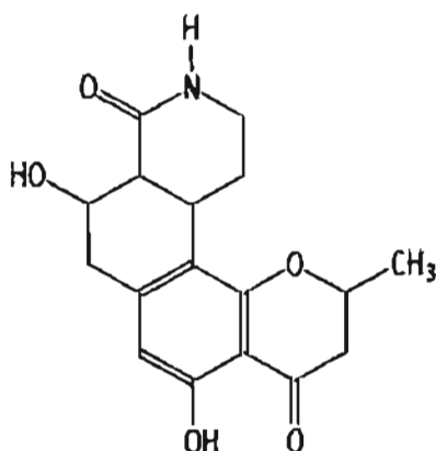
Figure 25 : Structure de la Schumannificine [105]
