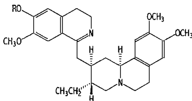
Figure 21 : Structure de la Psychotrine (R=H) et de l'O-Méthylpsychotrine (R=CH 3 ) [99]
