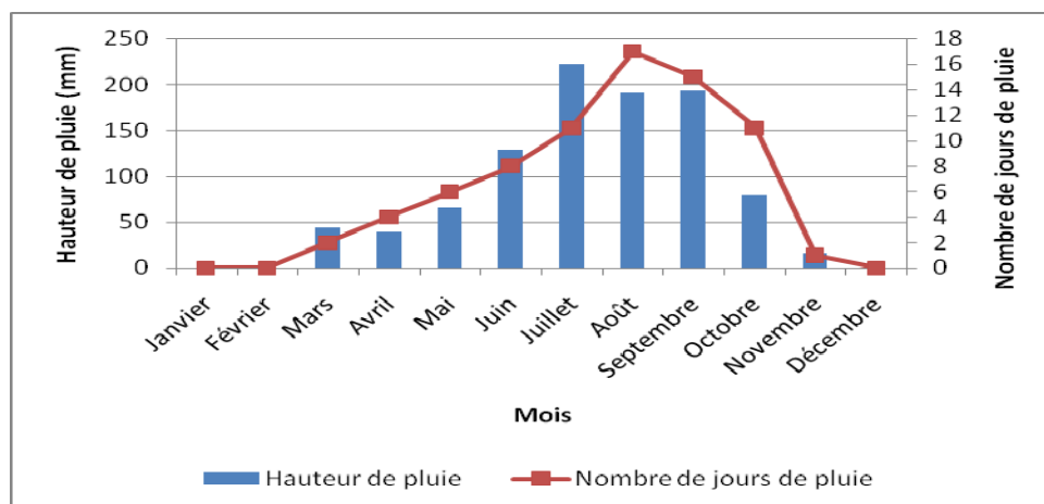
Figure 6 : Pluviosité de la station de Orodara durant l’année 2009
