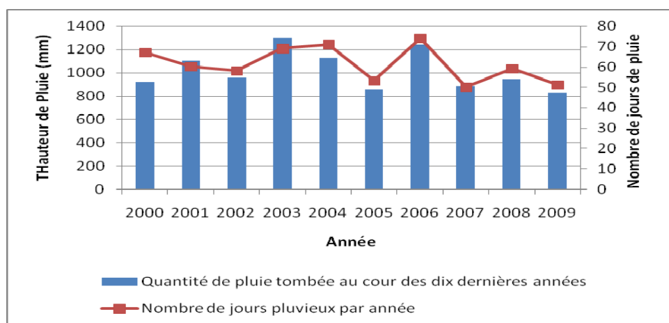
Figure 7 : Pluviométrie de la station de Mangodara au cours des dix dernières années
