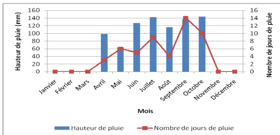
Figure 8 : Pluviométrie de la station de Mangodara durant l'année 2009
