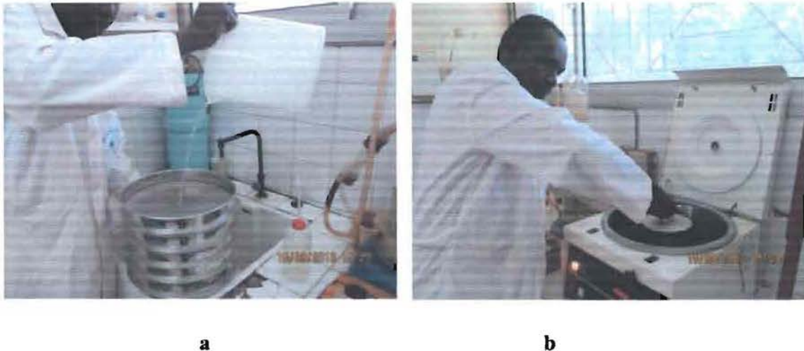
Figure 5 : Tamisage humide des échantillons de sol (a), récupération des échantillons après centrifugation (b)
