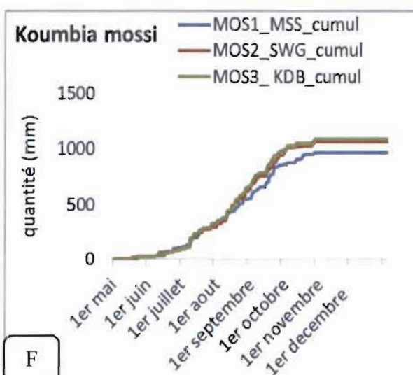
Figure 16: pluviométrie de chaque village par pluviomètre (2015)
